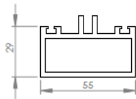
Onderprofiel 5529
