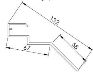
Montageprofiel
