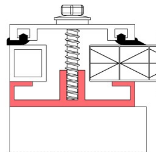
randprofiel
