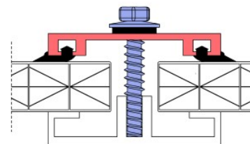
verbindingsprofiel
