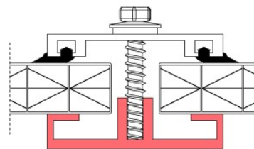
verbindingsprofiel
