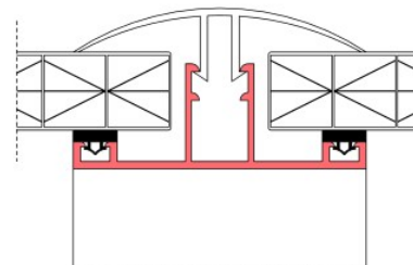
verbindingsprofiel
