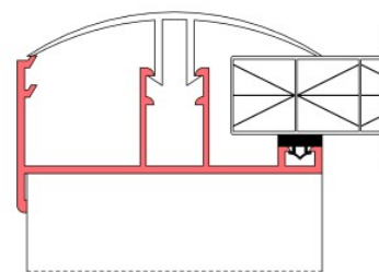
randprofiel
