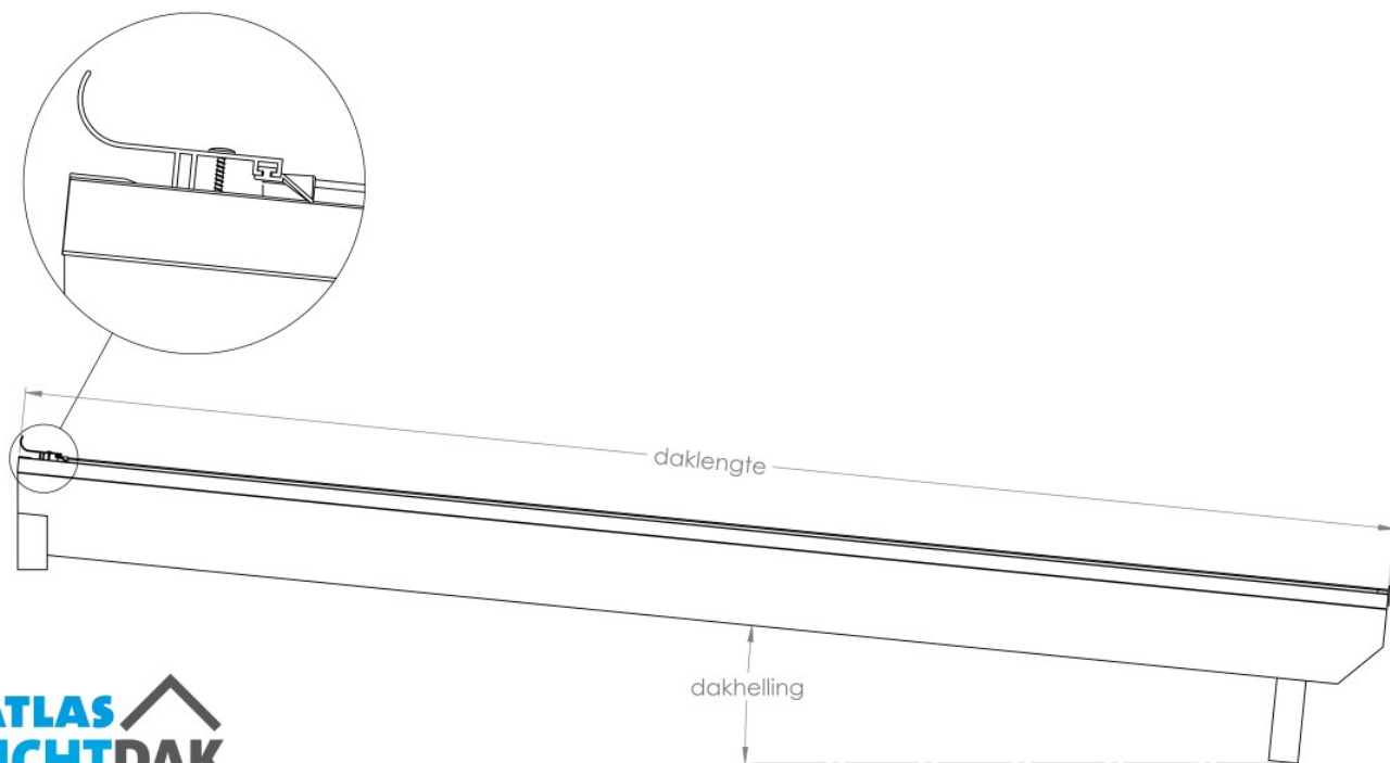
Onderdelen Atlas Lichtdak BASIC PC16
