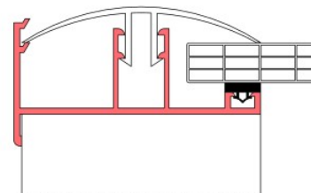
randprofiel
