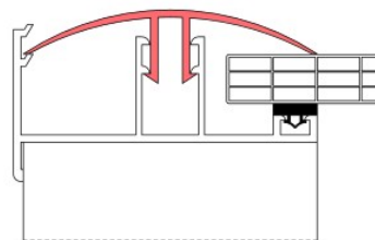
randprofiel
