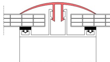
verbindingsprofiel
